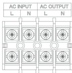
Клеммный блок
