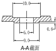
A-A截面
