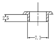
B-B截面
