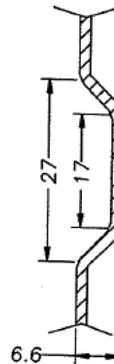
СЕЧЕНИЕ А—А МАСШТАБ: 4:1
