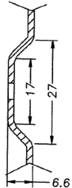
СЕЧЕНИЕ А—А МАСШТАБ: 4:1
